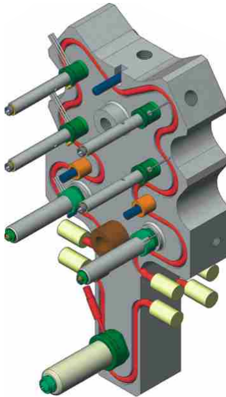
Das Bild zeigt ein 3D-Modell eines komplexen mechanischen Bauteils, das aus mehreren zylindrischen Komponenten und farbigen Schläuchen besteht.
